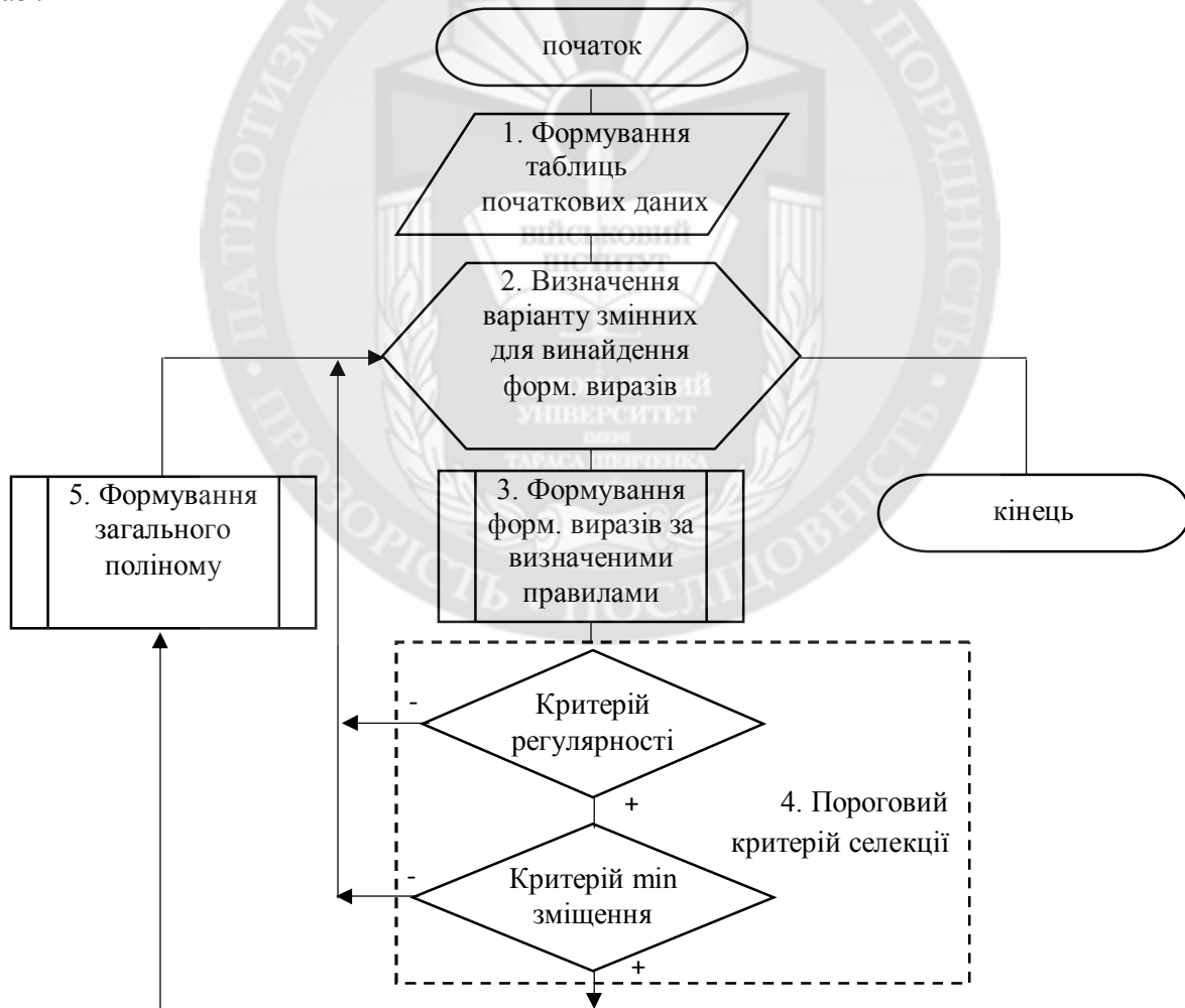
Рис. 2. Схема алгоритму побудови моделі складної системи з використанням комбінаторного методу з обмеженою базою аргументів
