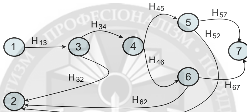
Рисунок 3 - Імовірнісний граф дій при виконанні захоплення обладнання оператора нелегітимним кореспондентом другого рівня
